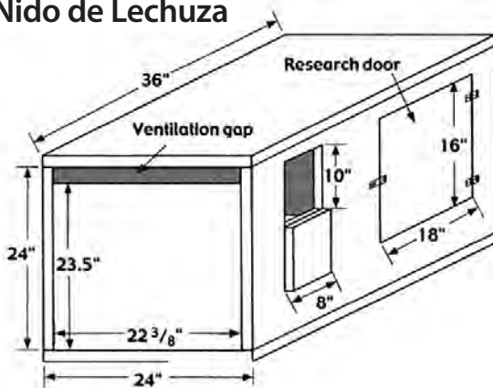
Diseño de caja de búhos. Ilustración: https://thebirdersreport.com/resources/nest-box-birdhouse-plans
